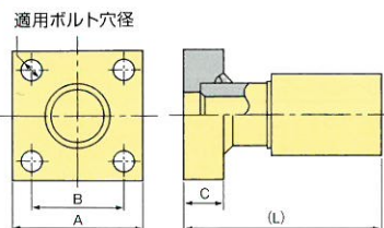
JIS B 2291 20.5MPa管フランジ
