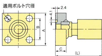
JIS B 2291 20.5MPa管フランジ
