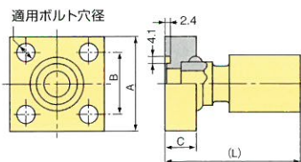
JIS B 2291 20.5MPa管フランジ
