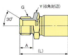
管用平行雄ねじ
