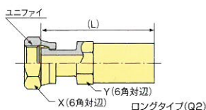
ユニファイ ロングタイプ(Q2)
