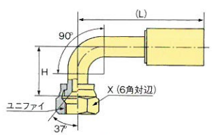
ユニファイ雌ねじ90° ベンド (雌37° シート)
