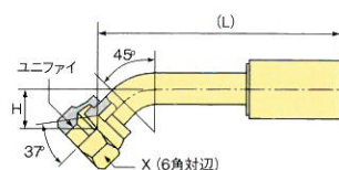
ユニファイ雌ねじ45° ベンド (雌37° シート)
