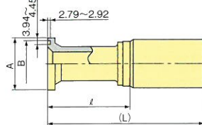
フランジタイプ(SAEスタンダード用)
