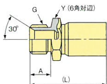
管用平行雄ねじ
