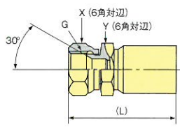
管用平行雌ねじ (雌30° シート)
