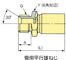
管用平行雄ねじ
