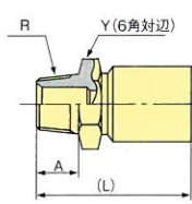
管用テーパ雄ねじ
