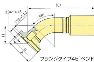
フランジタイプ45°ベンド (SAEスタンダード用)
