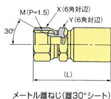
メートル雌ねじ(雌30°シート)
